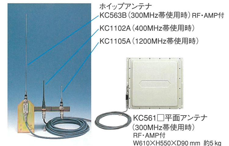
受信装置 KC211□B/KC212□B W360×H605×D215 mm (突起部除く) 約20kg以下
